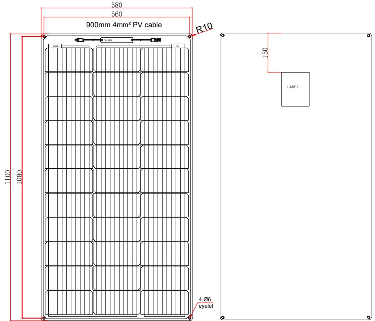
LE-M2-120W
